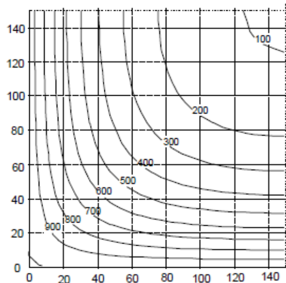
A13. ábra: Hőmérséklet-eloszlás (°C) oszlopban, h \times b = 300 \times 300 mm, R 90
