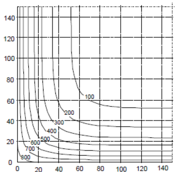
A11. ábra: Hőmérséklet-eloszlás (°C) oszlopban, h \times b = 300 \times 300 mm, R 30
