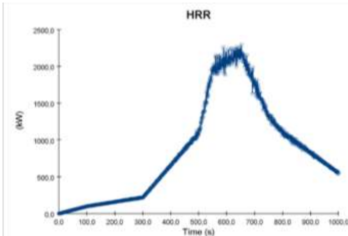
Széktűz HRR görbéje
