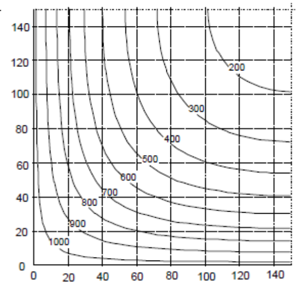
A14. ábra: Hőmérséklet-eloszlás (°C) oszlopban, h \times b = 300 \times 300 mm, R 120
