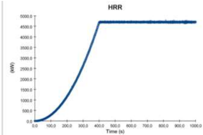
Színpadtűz HRR görbéje
